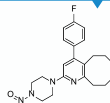
N-Nitroso desethyl Blonanserin
