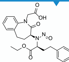
N-Nitroso Benazepril
