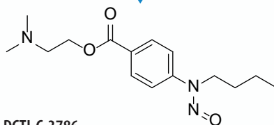
N-nitroso-tetracaine
