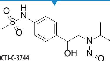
N-Nitroso-Sotalol
