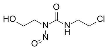
3-(2-chloroethyl)-1-(2-hydroxyethyl)-1-nitrosourea
