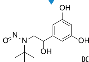
N-Nitroso Terbutaline
