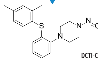
N-Nitroso-Vortioxetine
