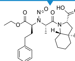
N-nitroso-trandolapril
