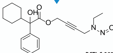
N-Nitroso N-Desethyl Oxybutynin
