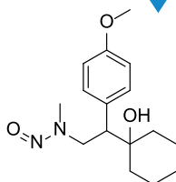
N-desmethyl-n-nitroso venlafaxine
