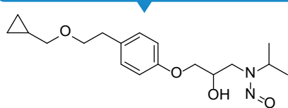
N-Nitroso-Betaxolol
