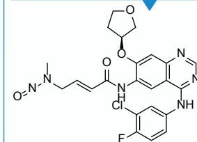
N-desmethyl-N-nitroso Afatinib
