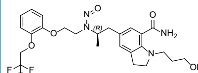
N-Nitroso Silodosin
