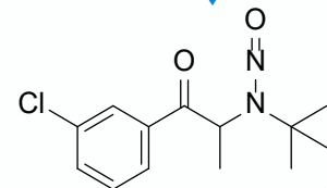
N-Nitroso Bupropion
