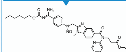
N-Nitroso Dabigatran etexilate
