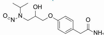
N-Nitroso Atenolol Impurity
