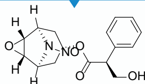
N-Nitroso Scopolamine
