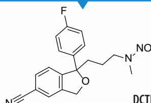
N-Nitroso Citalopram
