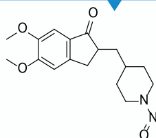
N- Nitroso Donepezil EP Impurity A
