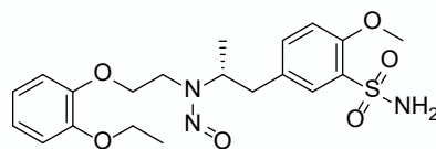
N-Nitroso Tamsulosin Impurity
