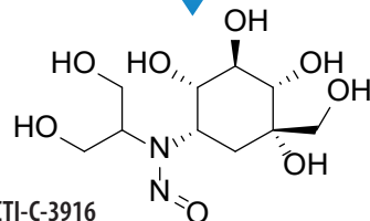
N-Nitroso Voglibose impurity
