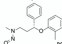
N-Nitroso atomoxetine
