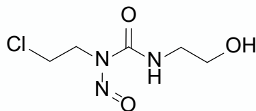
1-(2-chloroethyl)-3-(2-hydroxyethyl)-1-nitrosourea
