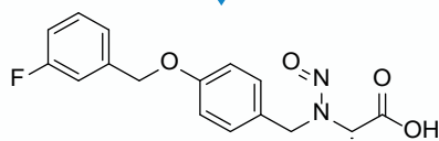
N-(4-((3-fluorobenzyl)oxy)benzyl)-N-nitroso-L-alanine
