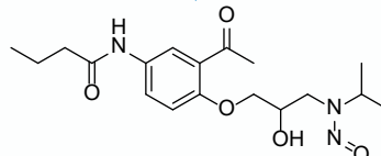
N-Nitroso-Acebutolo
