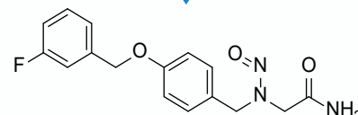
N-Nitroso-Safnamide
