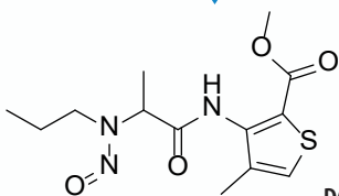
N-nitroso-Articaine
